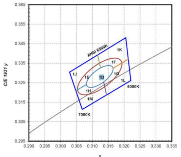
Abbildung 6: MacAdam 3 SDCM Ellipse mit ANSI °K Angaben. Die Tangenten zur schwarzen Körperkurve entsprechen den jeweiligen Farbttemperaturen.
