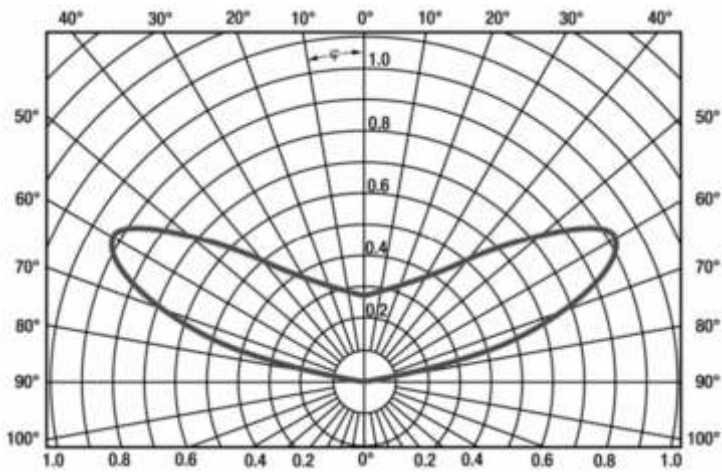
Abbildung 5: Relative Lichtverteilung I_v/I_{max} in (%)
