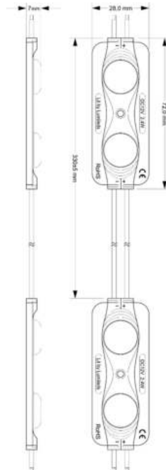
Abbildung 2: Moduldimensionen
